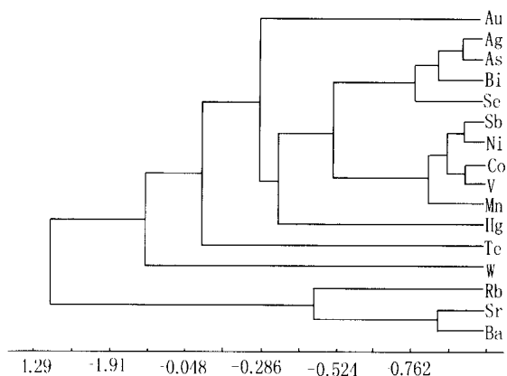
图2 金矿石微量元素 R 型聚类分析图谱
