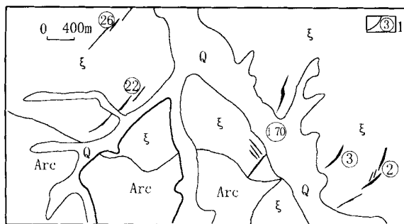
图 1 东坪金矿床地质简图
