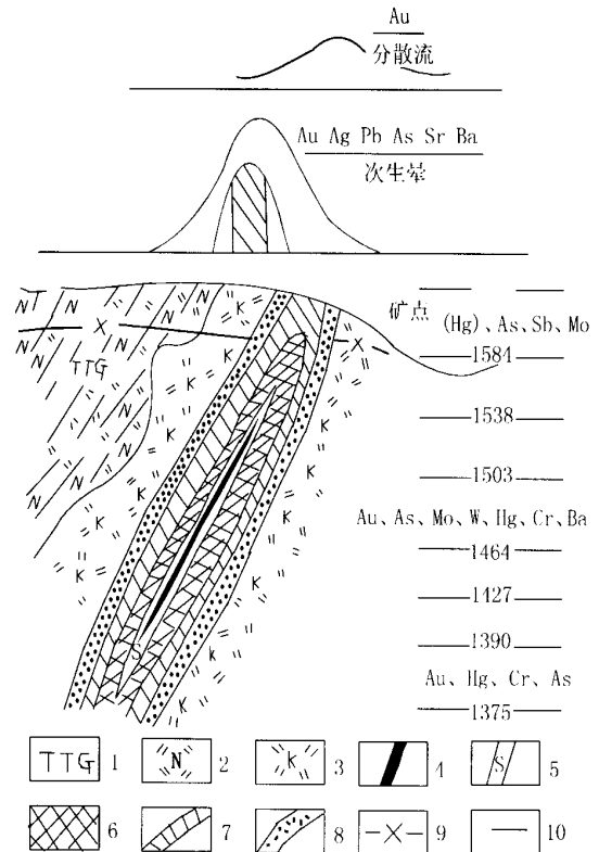
图 3 东坪金矿床地质—地球化学找矿模型
