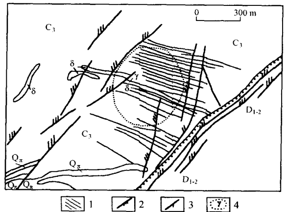
图1 大吉山钽铌钨矿地质略图 (据《大吉山钽铌钨矿勘探报告》修编)
