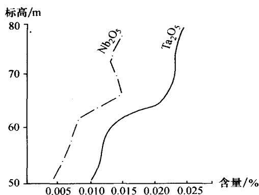
图 3 CK90 钽铌含量垂向变化曲线图 (据《大吉山钽铌钨矿勘探报告》修编)
