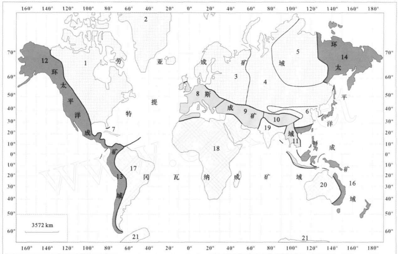
图 1 全球成矿单元划分略图
