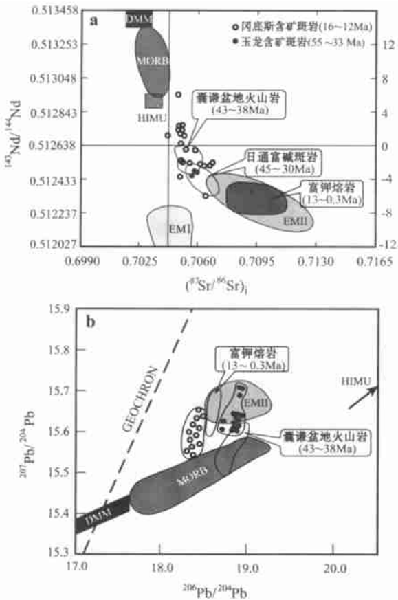
图 6 青藏高原含矿斑岩的 Sr-Nd-Pb 同位素特征图 a. ^{87}\text{Sr}/^{86}\text{Sr} - ^{143}\text{Nd}/^{144}\text{Nd} 图; b. ^{207}\text{Pb}/^{204}\text{Pb} - ^{206}\text{Pb}/^{204}\text{Pb} 图,显示青藏高原含矿斑岩的同位素地球化学特征。DMM, HIMU, EM 和 EM 分别代表 4 种地幔端元 (Zindle et al., 1986)。DMM: 亏损的 MORB 地幔; HIMU: 长期高 U/Pb 地幔; EM : 类型 富集地幔; EM : 类型 富集地幔; 玉龙斑岩带 Sr-Nd 同位素资料来自王增等(1995)和张玉泉等(1998a); 铅同位素资料来自马鸿文(1990); 日通富碱斑岩及囊谦盆地火山岩同位素资料来自 Sun 等(2001); 冈底斯斑岩带 Sr-Nd、Pb 同位素资料来自侯增谦和曲晓明未刊资料
