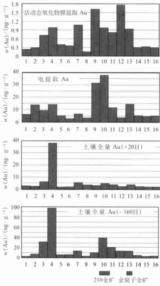
图 13 3 种方法在中国金窝子金矿上方对比结果
