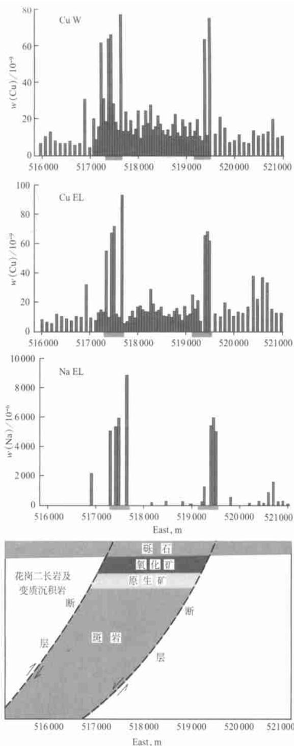
图 10 Actlabs 水提取及酶提取在 Gaby Sur 矿沿两侧断层在地表呈现的 Cu 及 Na 的异常峰
