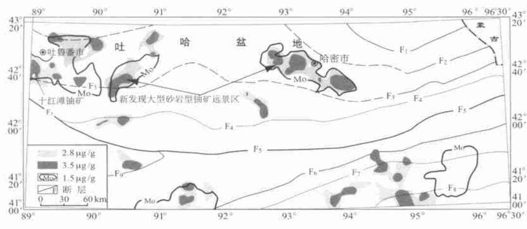
图 12 新疆东天山地区 U、Mo 的地球化学异常分布图
