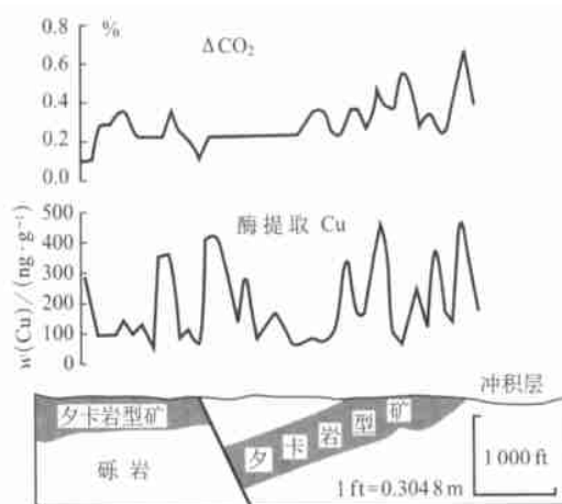
图 2 Ruby Star 夕卡岩型铜矿床 4600E 剖面上 \text{CO}_2 及酶提取圈定的 Cu 异常
