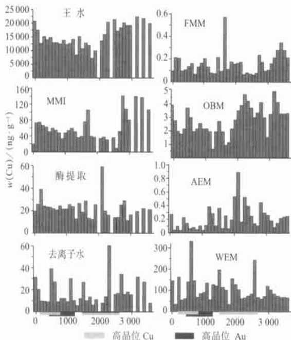
图 8 用各种分析方法分析活动态 Cu 的结果 Fig. 8 Comparison of mobile Cu variation over Mike deposit using different analytical methods
