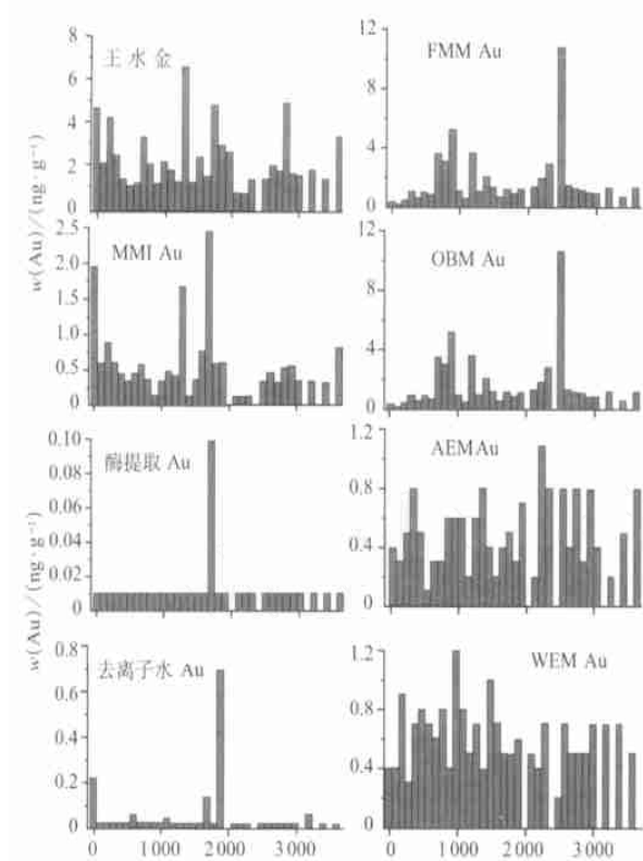
图 7 用各种方法分析 Mike 矿床上的活动态 Au 的结果 Fig. 7 Comparison of mobile Au variation over Mike deposit using different analytical
