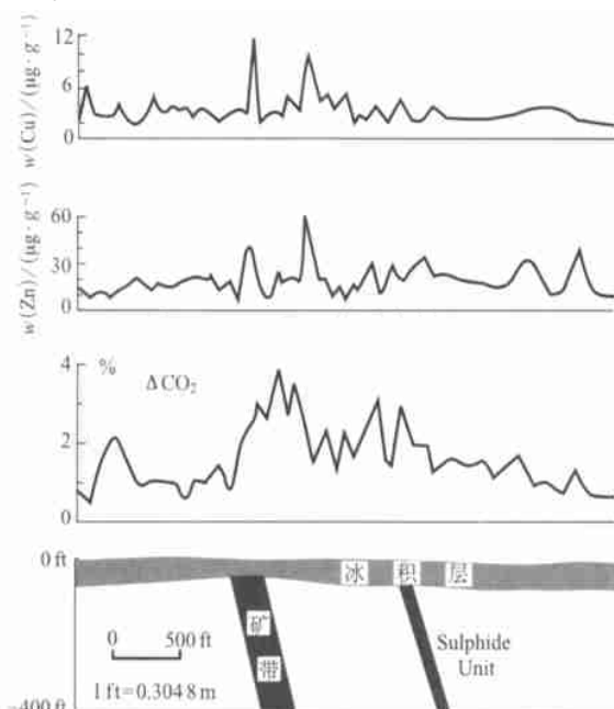
图 1 Crandon 块状硫化物矿床上方酶提取方法圈出的 \text{CO}_2 、Cu 及 Zn 异常
