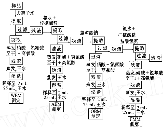
图 14 物化探所发展的活动态金属循序提取流程
