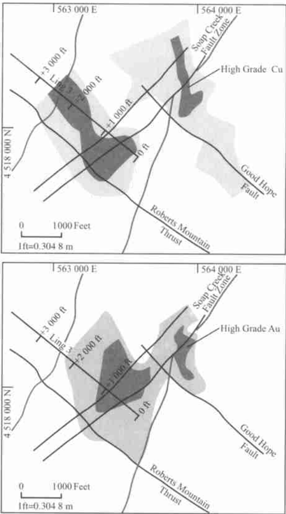
图 6 Mike 矿床的地质与矿化 Fig. 6 Geology and mineralization, Mike deposit
