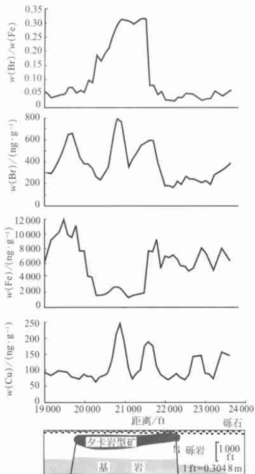
图3 Ruby Star 夕卡岩型矿床 32000N 剖面线上酶提取圈出的 Cu、Br/ Fe 异常及 Fe 的负异常 [12]
