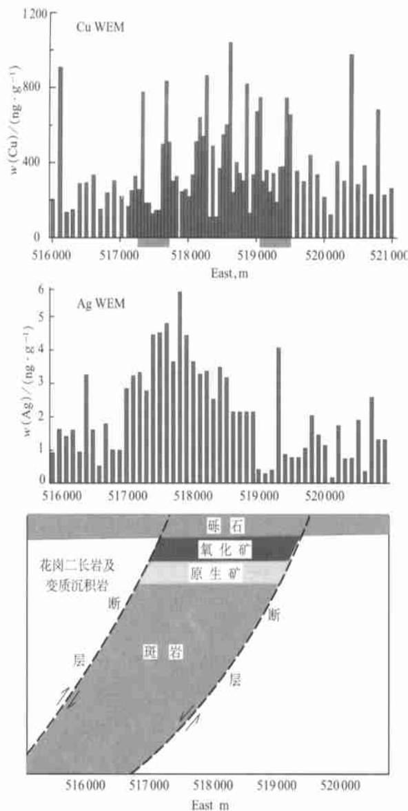
图 11 中国物化探所 WEM 提取在 Gaby Sur 矿床上方地表呈现的 Cu 及 Ag 异常
