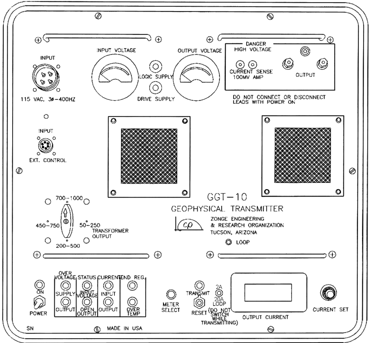
图 3. GGT-10, 前面板
