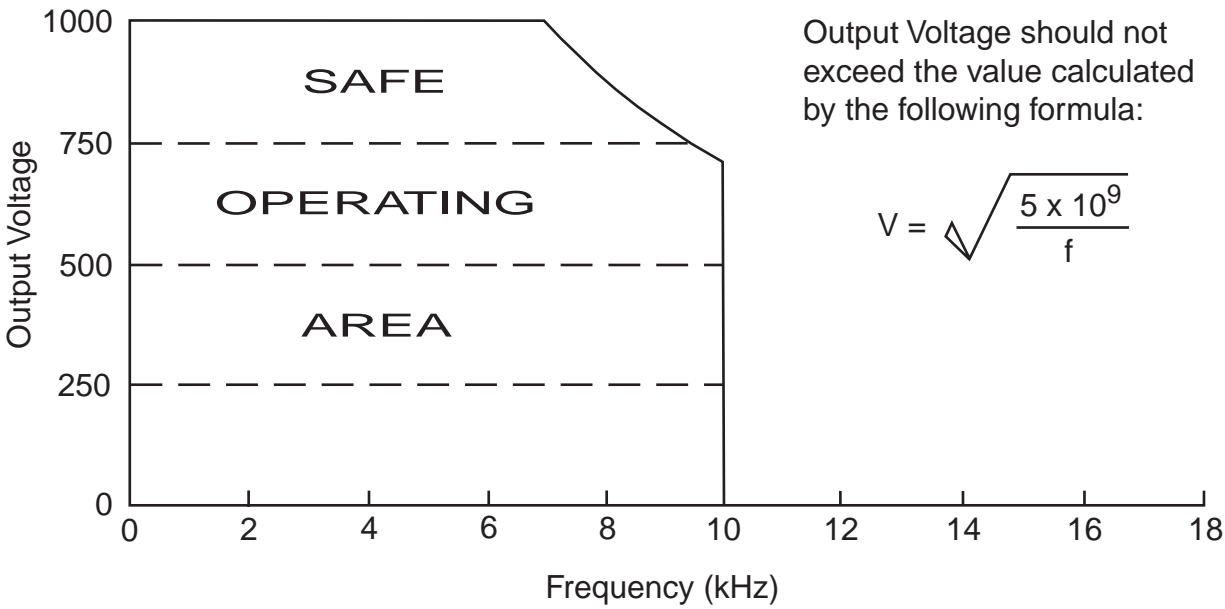
图 1. GGT-10 安全操作曲线
