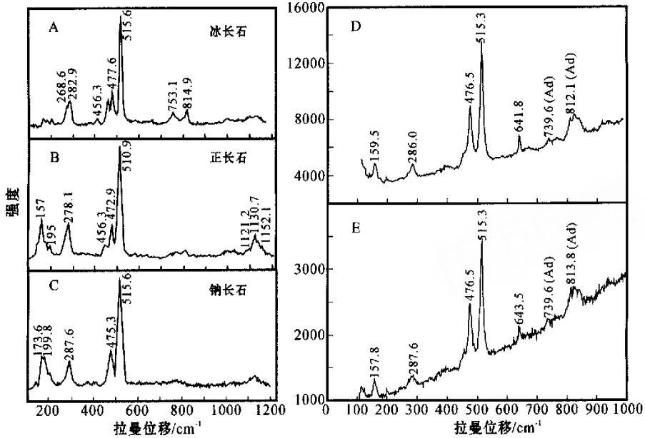
图3 祁雨沟含金角砾岩筒中的冰长石(Ad)与标准的冰长石、正长石和钠长石拉曼谱峰对比图
