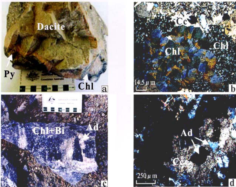
图5 绿泥石化和冰长石-碳酸盐化间的关系
