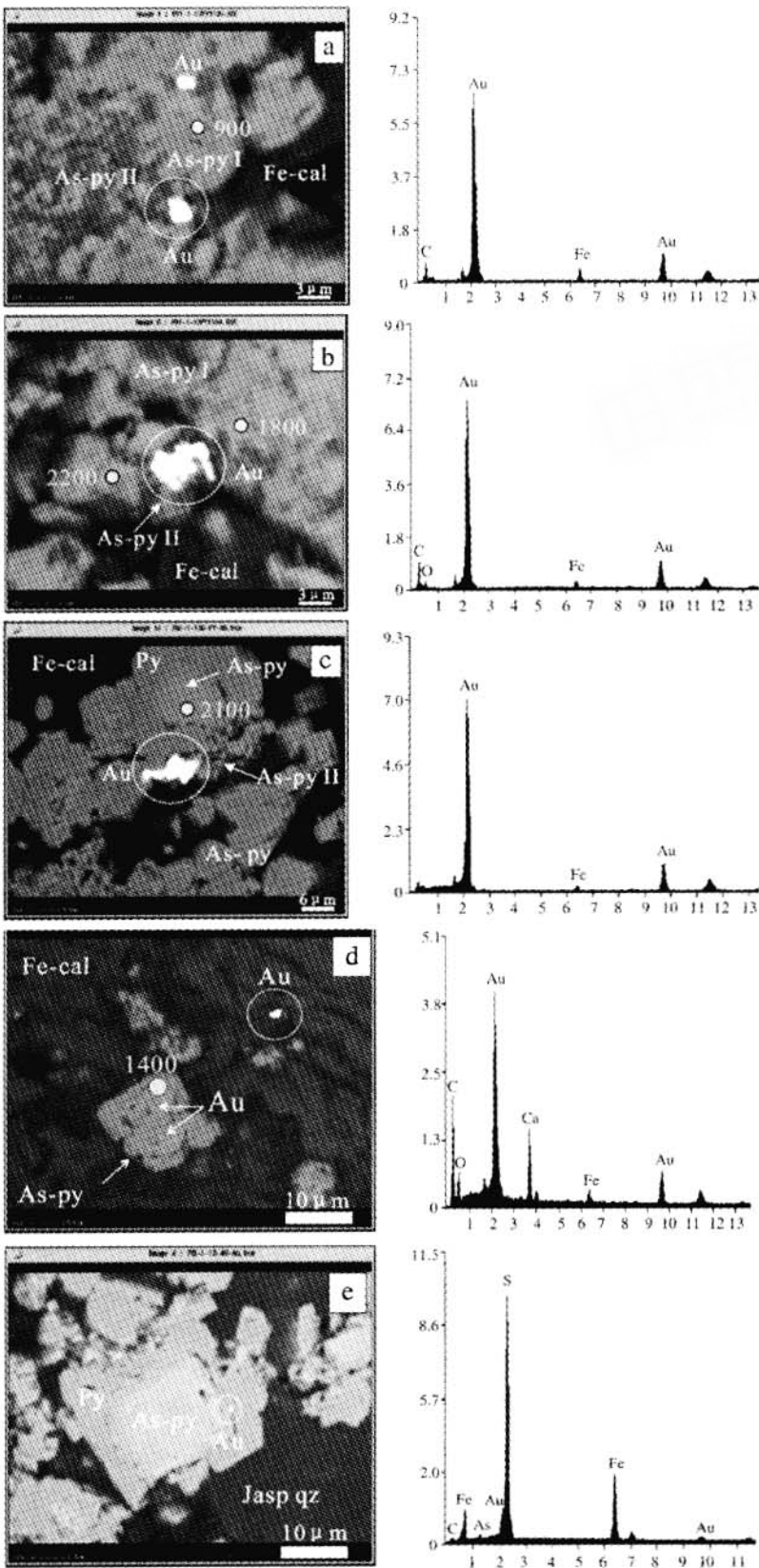
Fe-cal. 含铁方解石 As-py I. 早世代含砷黄铁矿 As-py II. 晚世代含砷黄铁矿 Au. 自然金颗粒 实心圆圈和数值分别示 WDS 分析的位置和金含量 ( \times 10^{-6} )
