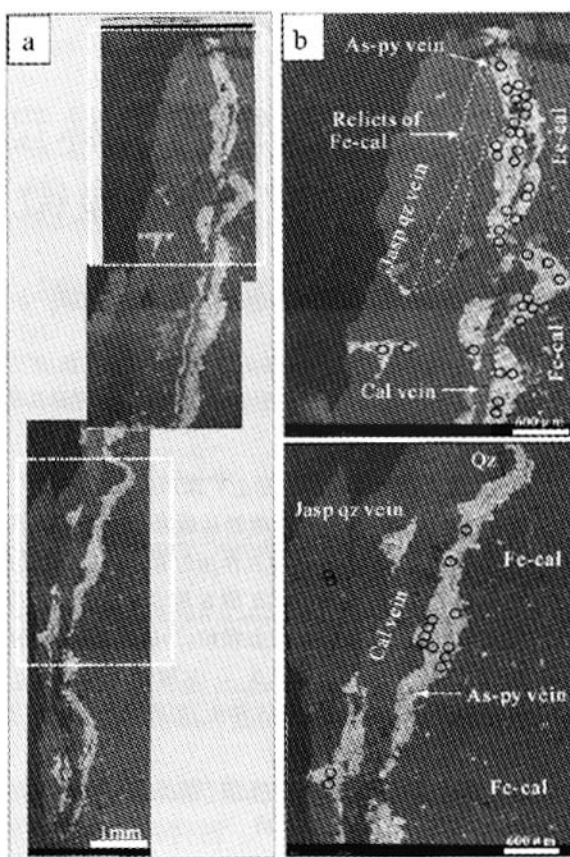
Jasp qz vein. 碧玉质石英脉 As-py vein. 含砷黄铁矿脉 Cal vein. 方解石脉 Fe-cal. 含铁方解石 空心圆图示自然金颗粒的位置
