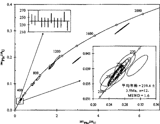
图 4 河台金矿混合岩锆石 U-Pb 谐和曲线图
