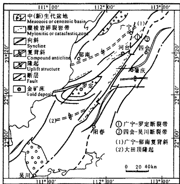
图 1 河台金矿床构造位置图
