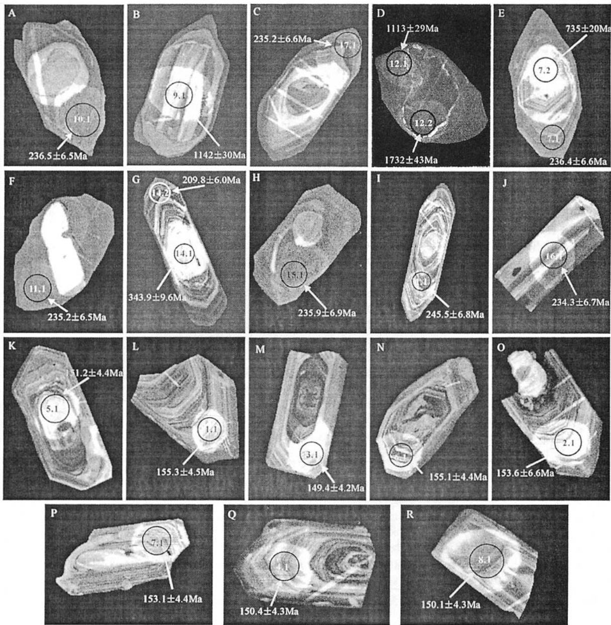
图 3 混合岩中锆石(A—J)及含金石英脉中锆石(K—R)阴极发光图像 (图中○圈出发亮位置为测点位置,○直径为 30 μm)
