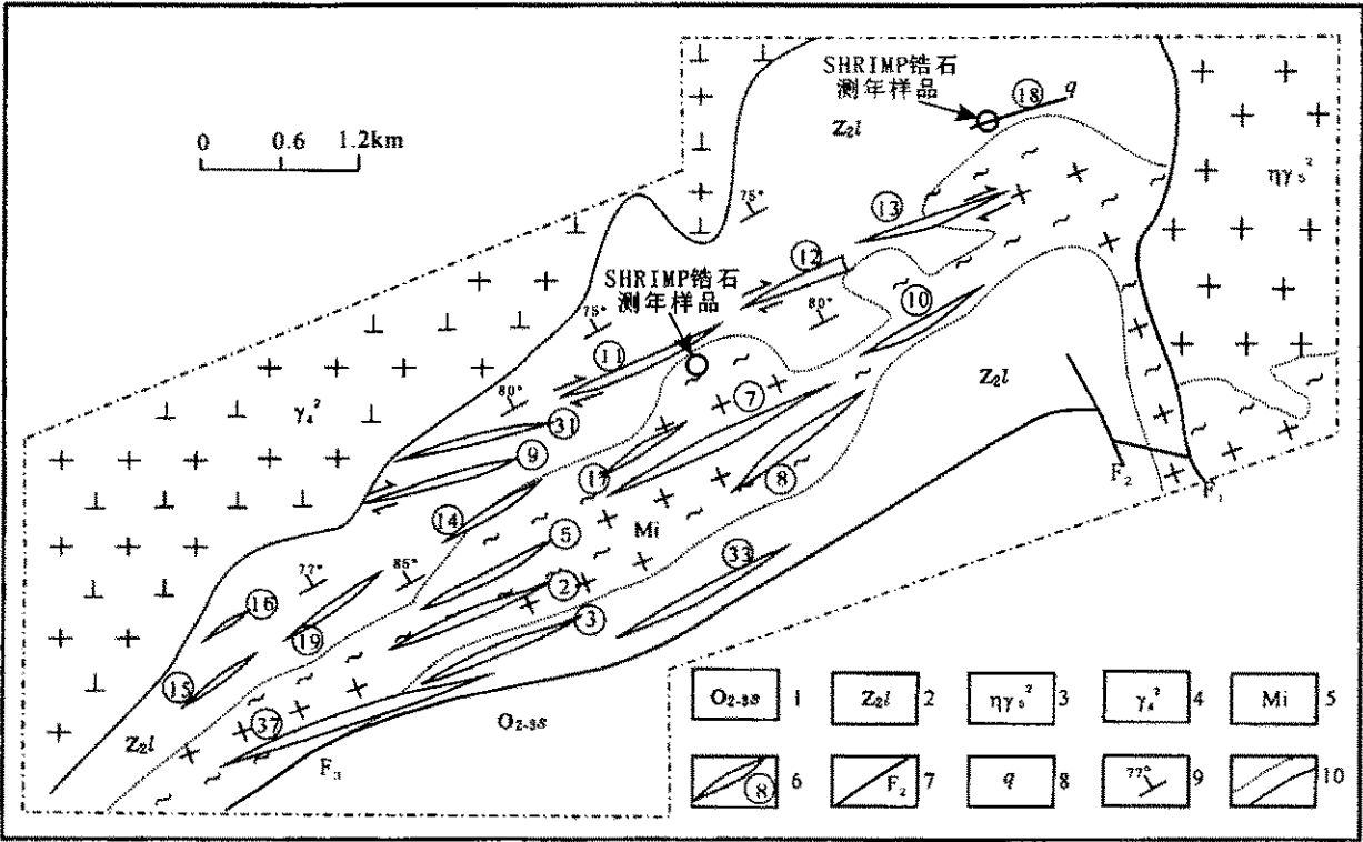
图 2 河台金矿床矿区地质及采样位置图(据广东省地矿局 719 地质大队 ® )
