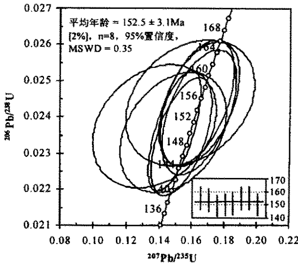
图 5 含金石英脉锆石 U-Pb 谐和曲线图
