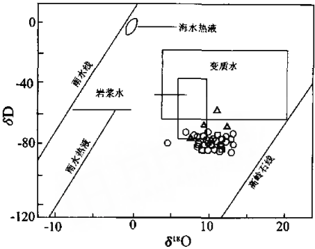
图4 八卦庙、李坝及小沟里金矿床石英氢氧同位素图
