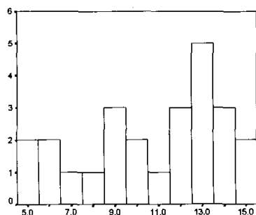
图 2 八卦庙金矿床矿石硫同位素频率分布直方图
