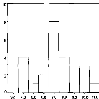
图 3 李坝金矿床矿石硫同位素分布直方图
